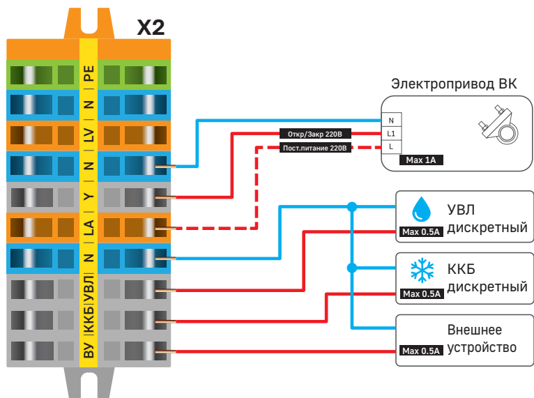
Рисунок 4. Схема подключения цепей AC230В.
