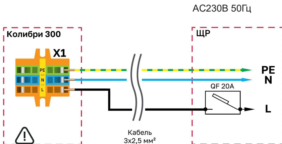
Рисунок 3. Схема подключения цепи питания AC230В 50Гц
